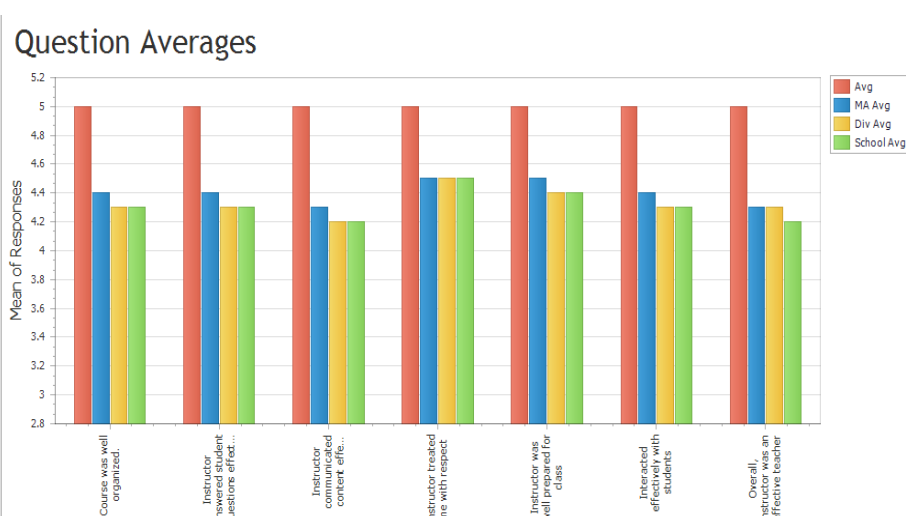
Calc 2, Fall 2016
